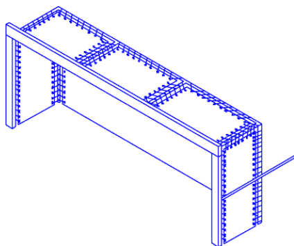
modèle fixé
